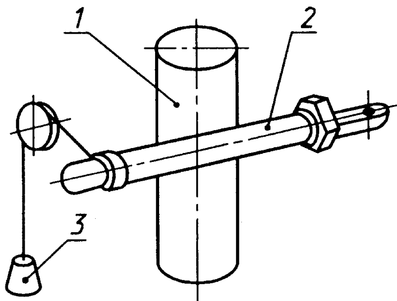
1 — рукав, 2 — калильный стержень, 3 — груз
