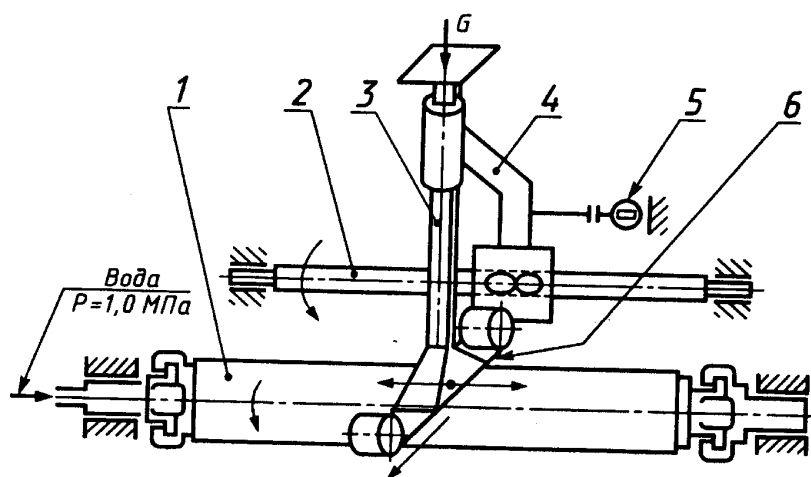
1 — рукав; 2 — вал привода суппорта; 3 — узел размещения и подачи абразивной ленты; 4 — суппорт; 5 — счетчик двойных ходов суппорта; 6 — абразивная лента
