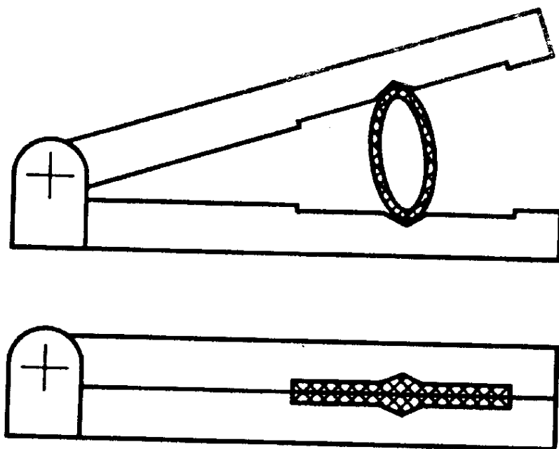
Рисунок А.3 — Приспособление для оценки морозостойкости рукава
